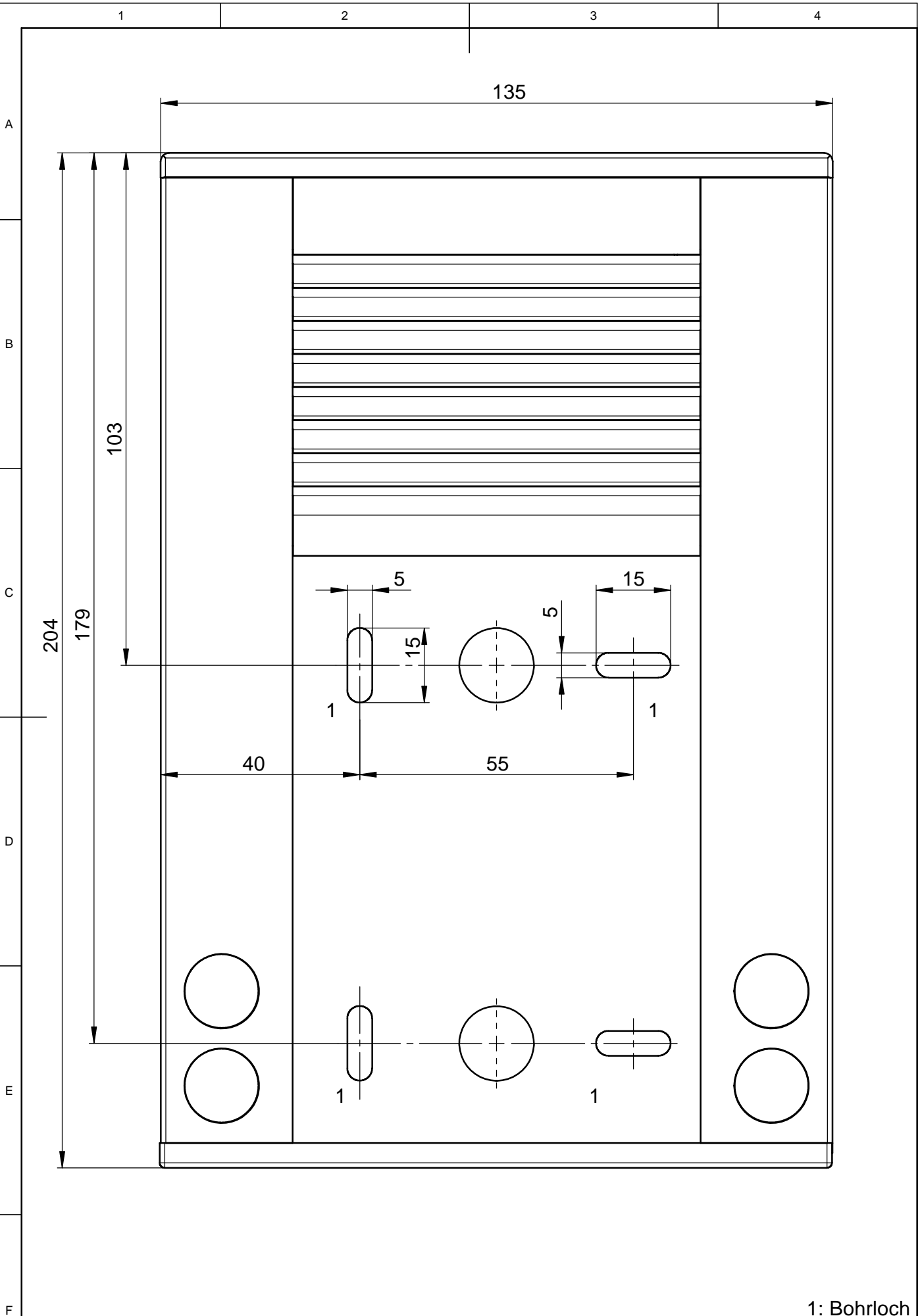
Bohrschablone ASE CS04
