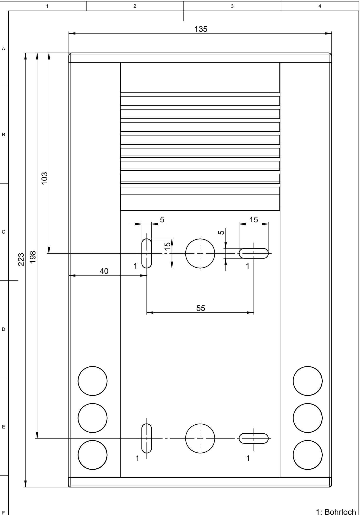
Bohrschablone ASE CS06
