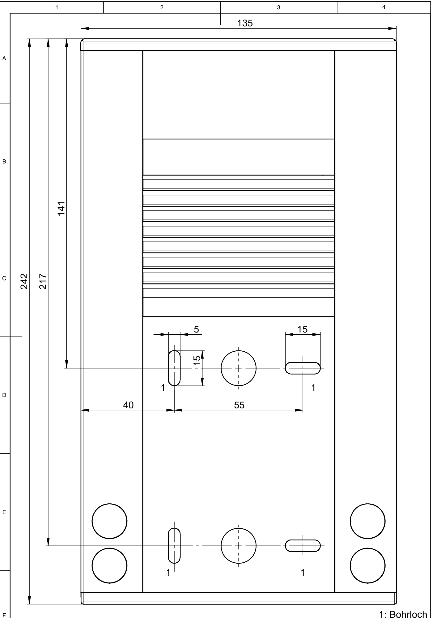
Bohrschablone AVE VCS04
