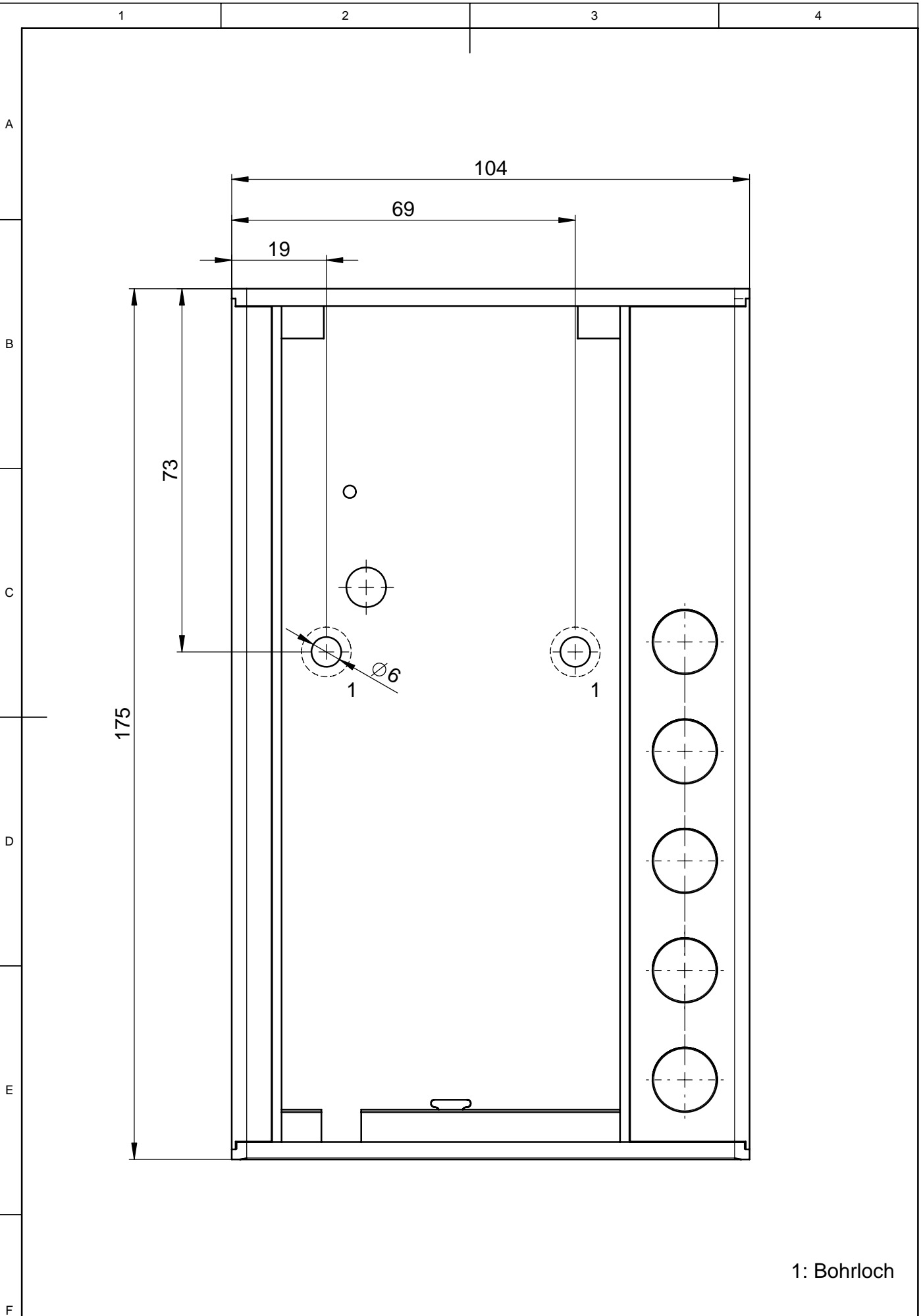
Bohrschablone PAK05
