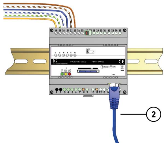
Abb. 5: Leitungen anschließen
