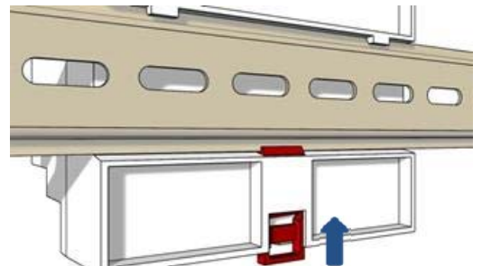
Abb. 2: Einrasten
