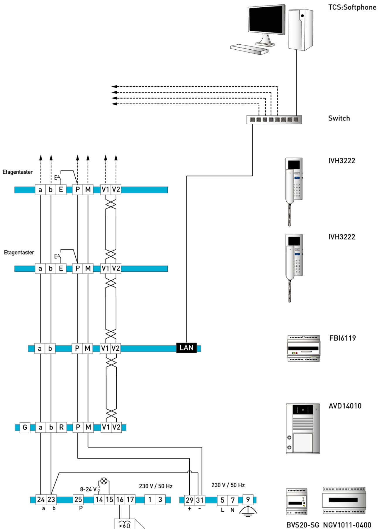
Abb. 6: Schaltungsbeispiel Basisinstallation
