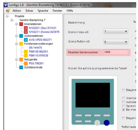
Abb. 46: Parallele Seriennummer ecoos und sky
