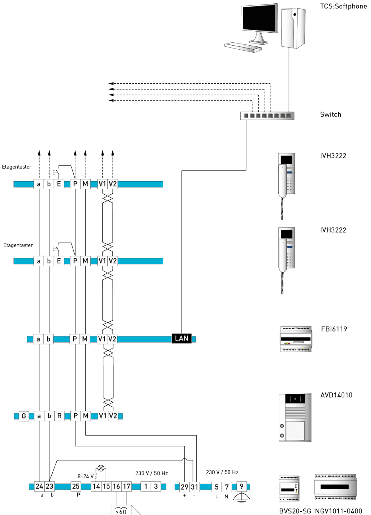
Abb. 6: Schaltungsbeispiel Basisinstallation
