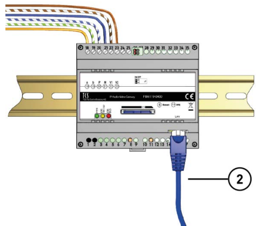
Abb. 5: Leitungen anschließen
