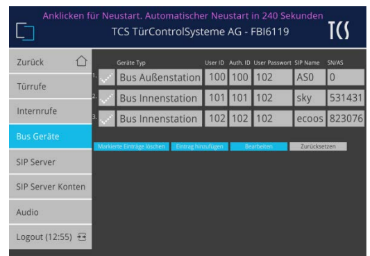
Abb. 51: Menü Bus Geräte
