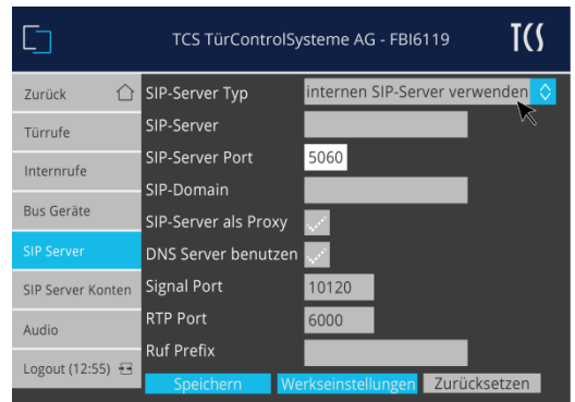
Abb. 27: Interner SIP-Server
