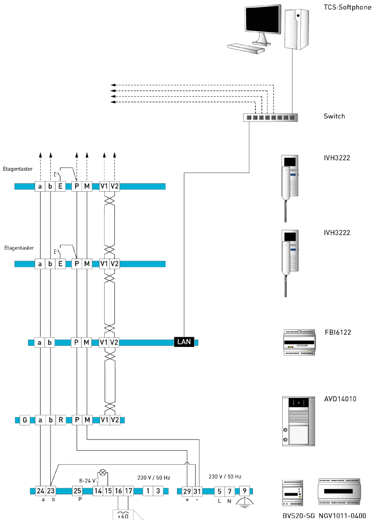
Abb. 6: Schaltungsbeispiel Basisinstallation
