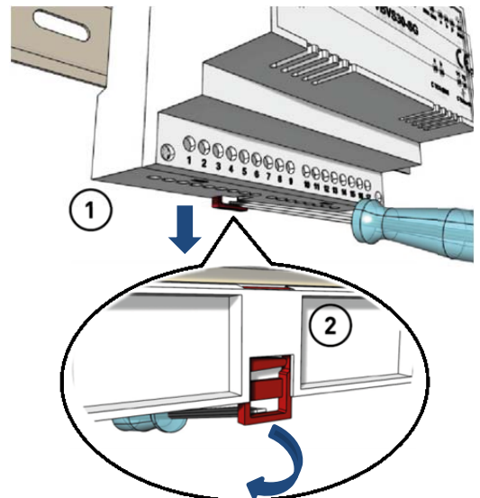
Abb. 3: von der Hutschiene demontieren
