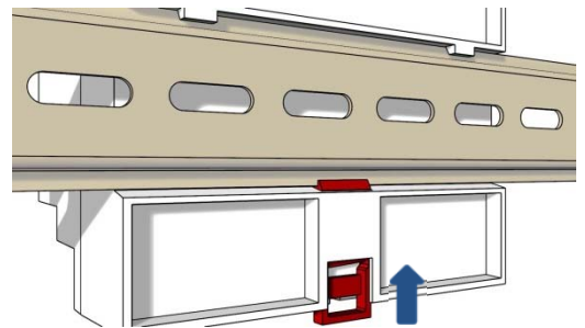
Abb. 2: Einrasten
