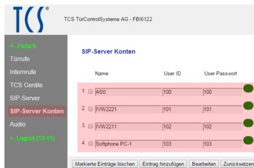
Abb. 49: SIP-Server Konten
