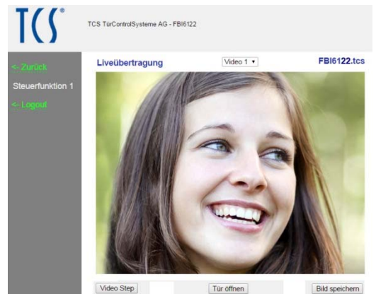
Abb. 19: Menü Liveübertragung
