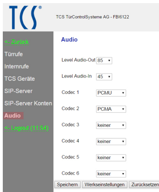
Abb. 28: Audio Einstellungen
