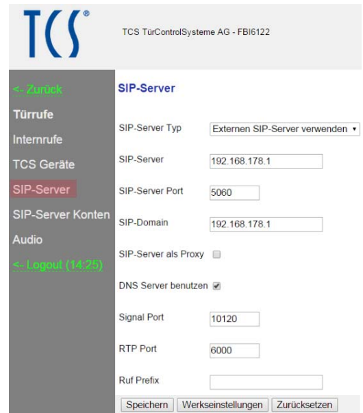
Abb. 63: SIP-Server
