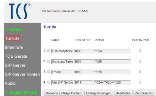
Abb. 23: Türrufe
