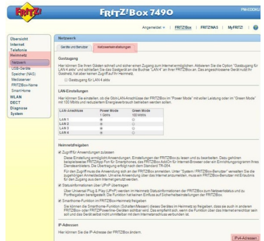
Abb. 54: Netzwerkeinstellungen
