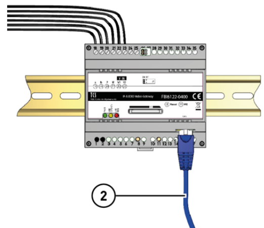
Abb. 5: Leitungen Anschließen
