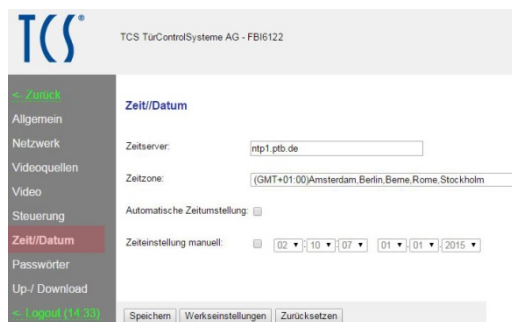
Abb. 35: Einstellungen Zeit/Datum
