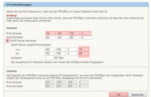
Abb. 55: IPv4-Einstellungen
