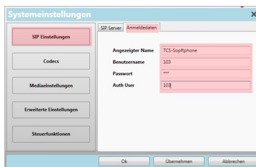
Abb. 51: Anmeldedaten
