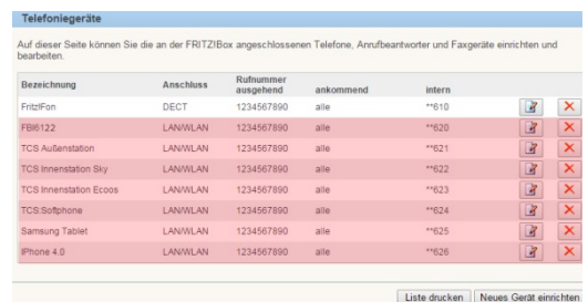
Abb. 60: Übersicht Telefoniegeräte
