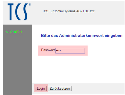
Abb. 62: Login
