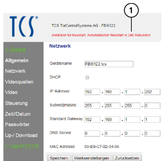
Abb. 17: Meldung Neustart
