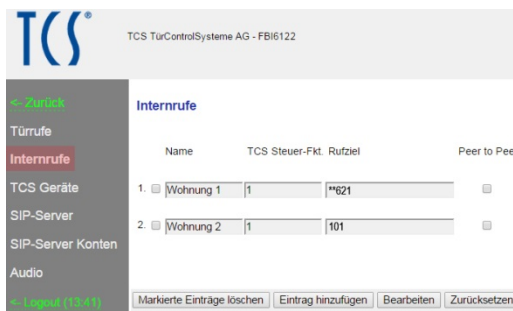
Abb. 24: Internrufe
