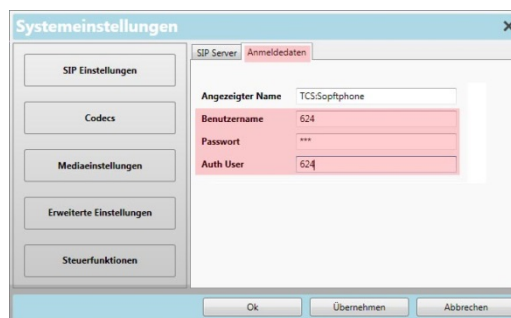
Abb. 67: Anmeldedaten
