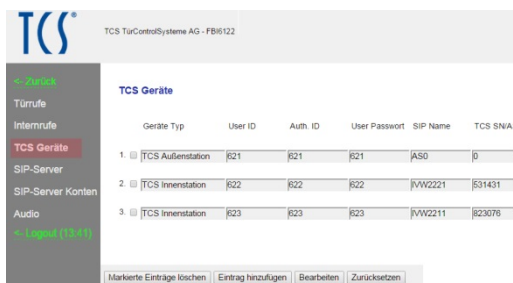
Abb. 25: TCS-Geräte
