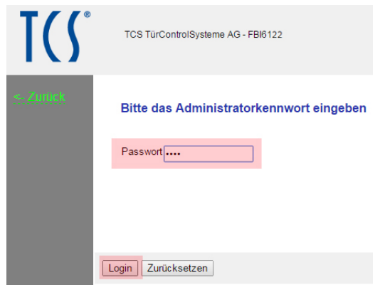
Abb. 45: Login
