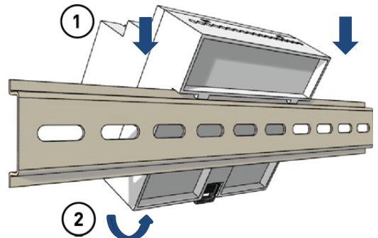
Abb. 1: Montage auf Hutschiene
