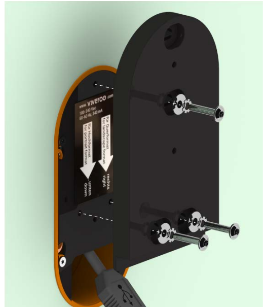
Abb. 7: Montageplatte befestigen
