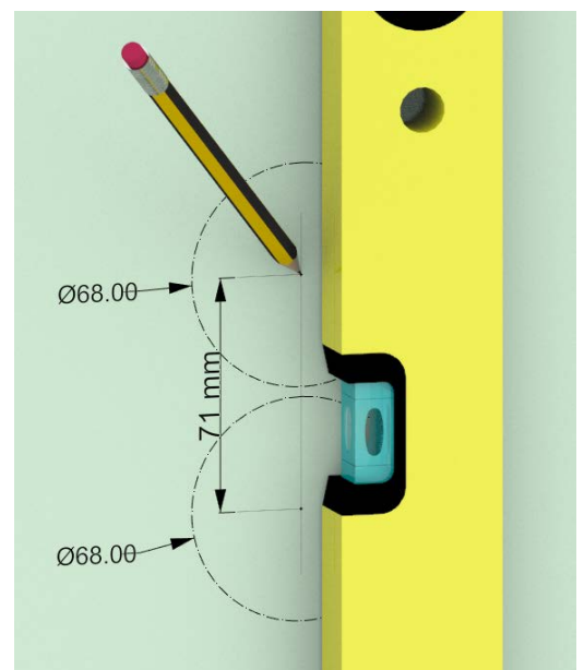
Abb. 4: Wandausschnitt anfertigen
