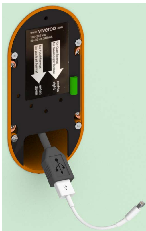
Abb. 6: Installationsträgerplatte montieren
