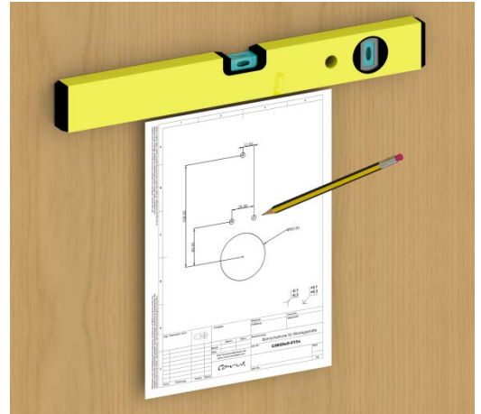
Abb. 1: Bohrschablone ausrichten
