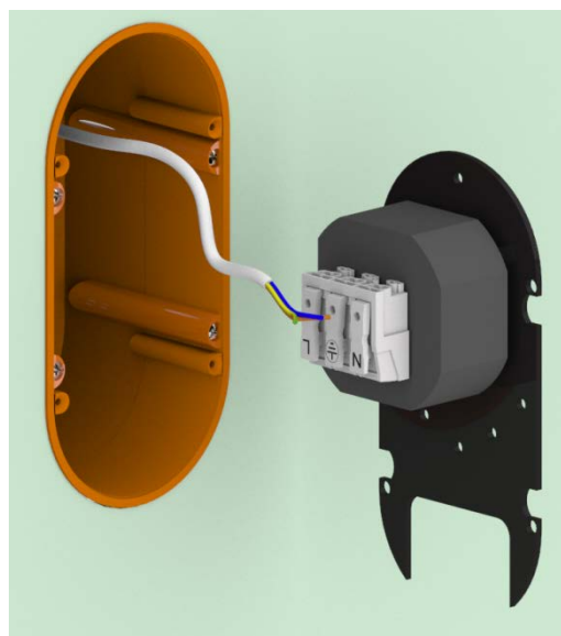
Abb. 5: Installationsträgerplatte befestigen
