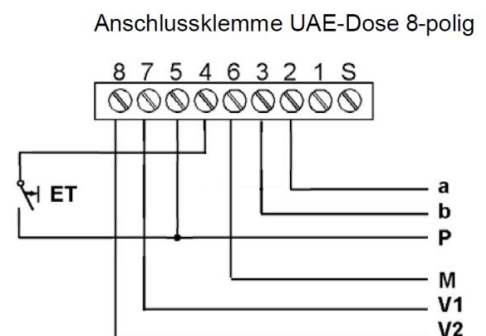
Abb. 1: Anschlussschema 6-Drahttechnik
