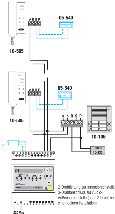
Abb. 4: vollständiger Anschlussplan
