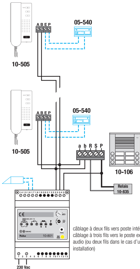
Fig. 4 : schéma de raccordement complet
