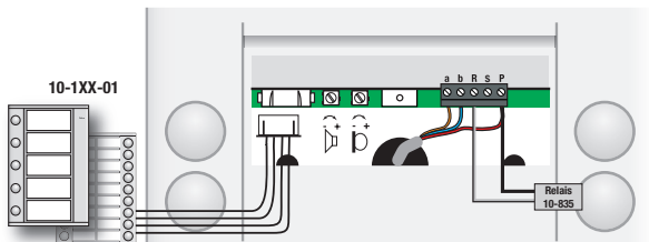
Obr. 3: pripojovacie svorky a ovládanie hlasitosti
