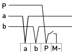
TCS:BUS-Klemmen, Eingangsklemmen
