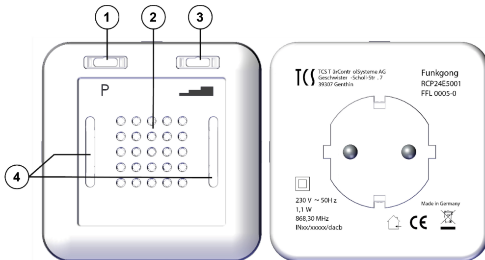
Abb. 1: Geräteübersicht
