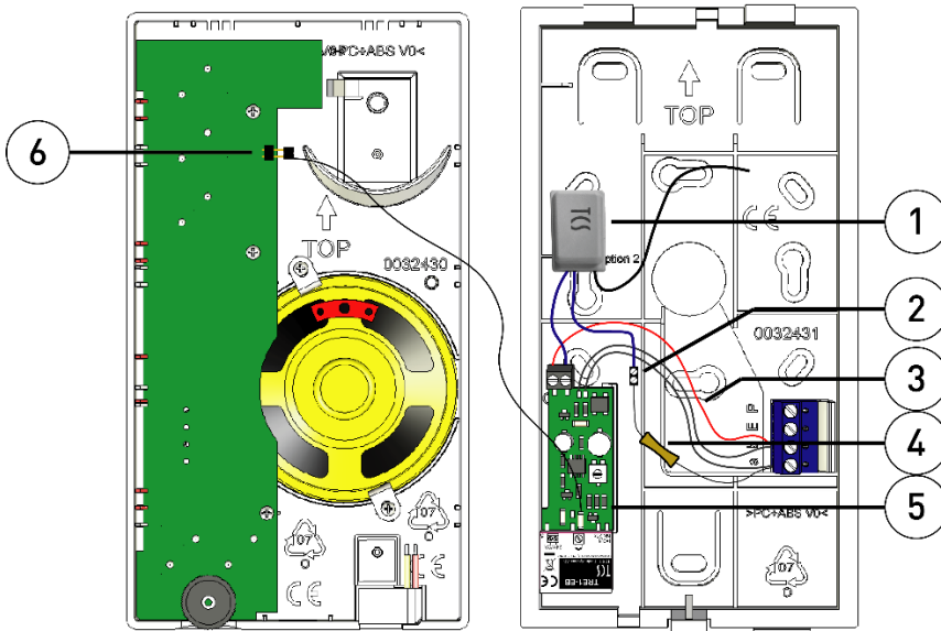
Abb. 2: Einbau RTS17E und TRE1-EB/1 und Anschluss in 2-Drahttechnik (am Beispiel ISH3030)
