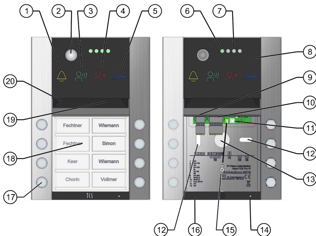
Abb. 1: Geräteübersicht
