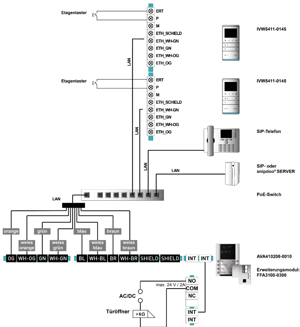
Abb. 10: Schaltungsbeispiel
