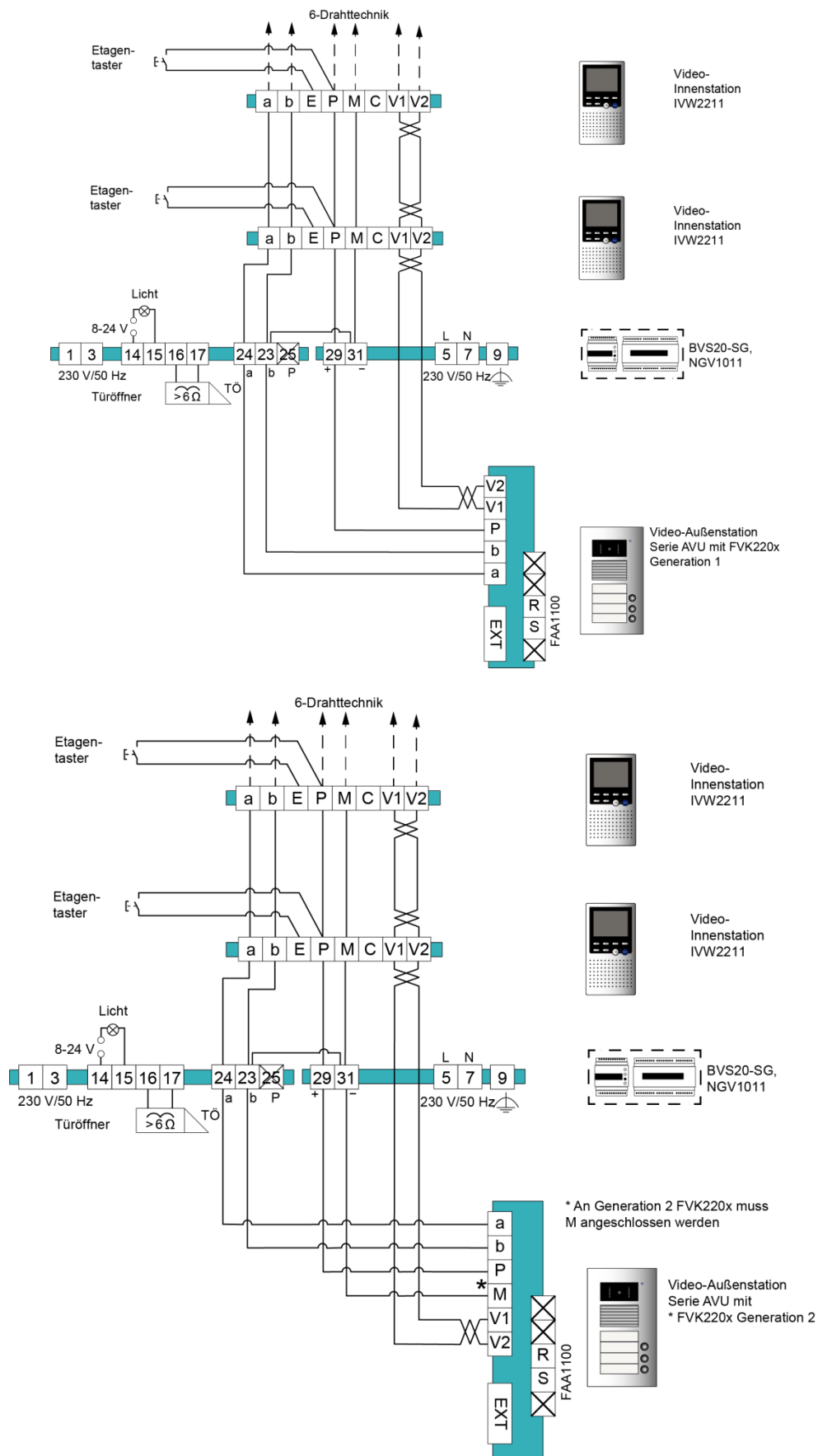
Abb. 5: Schaltungsbeispiele
