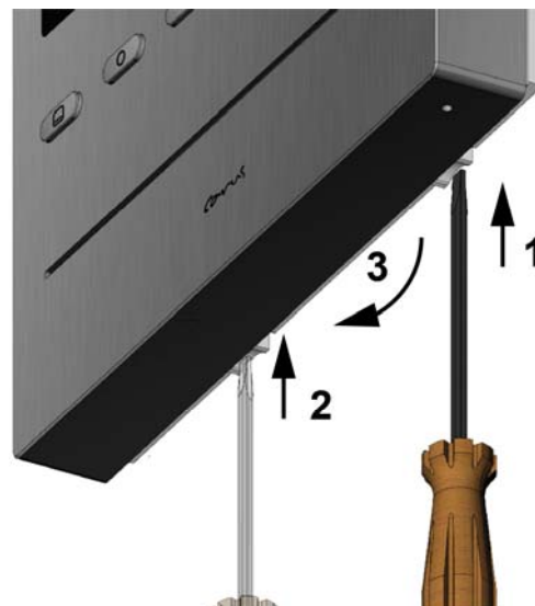
Abb. 8: Gerät auf die Unterschale aufrasten
