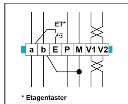
Abb. 5: 5-Drahttechnik
