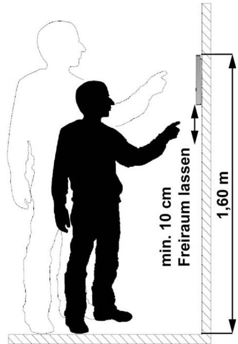
Abb. 2: Montagehöhe
