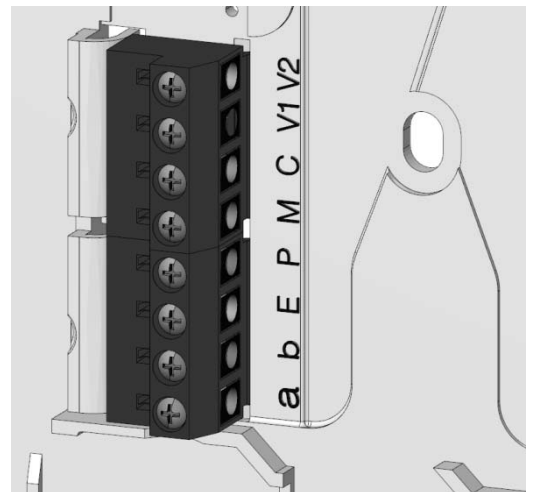
Abb. 4: Leitungen anschließen
