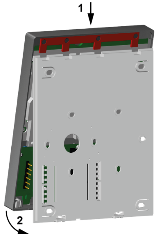
Abb. 7: Gerät auf die Unterschale aufrasten
