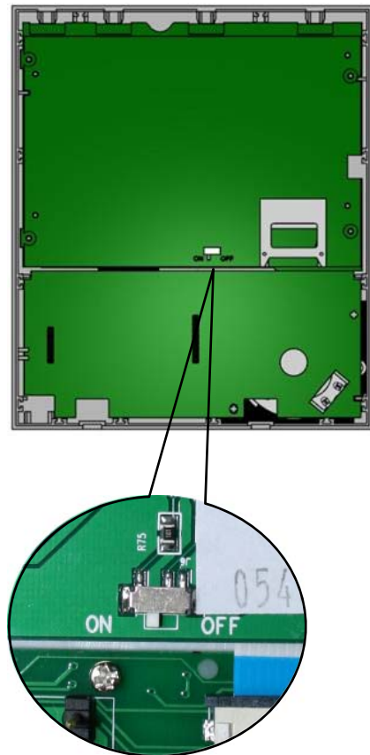
Abb. 6: Abschlusswiderstand
