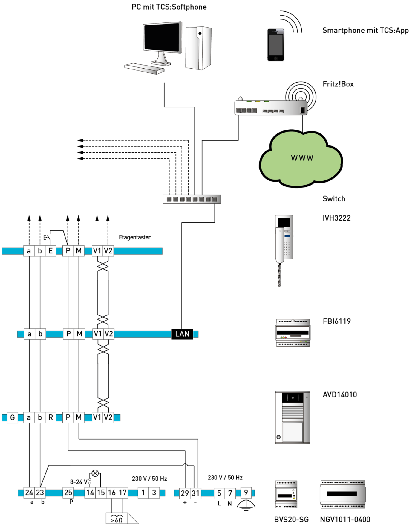
Abb. 6: Schaltungsbeispiel
