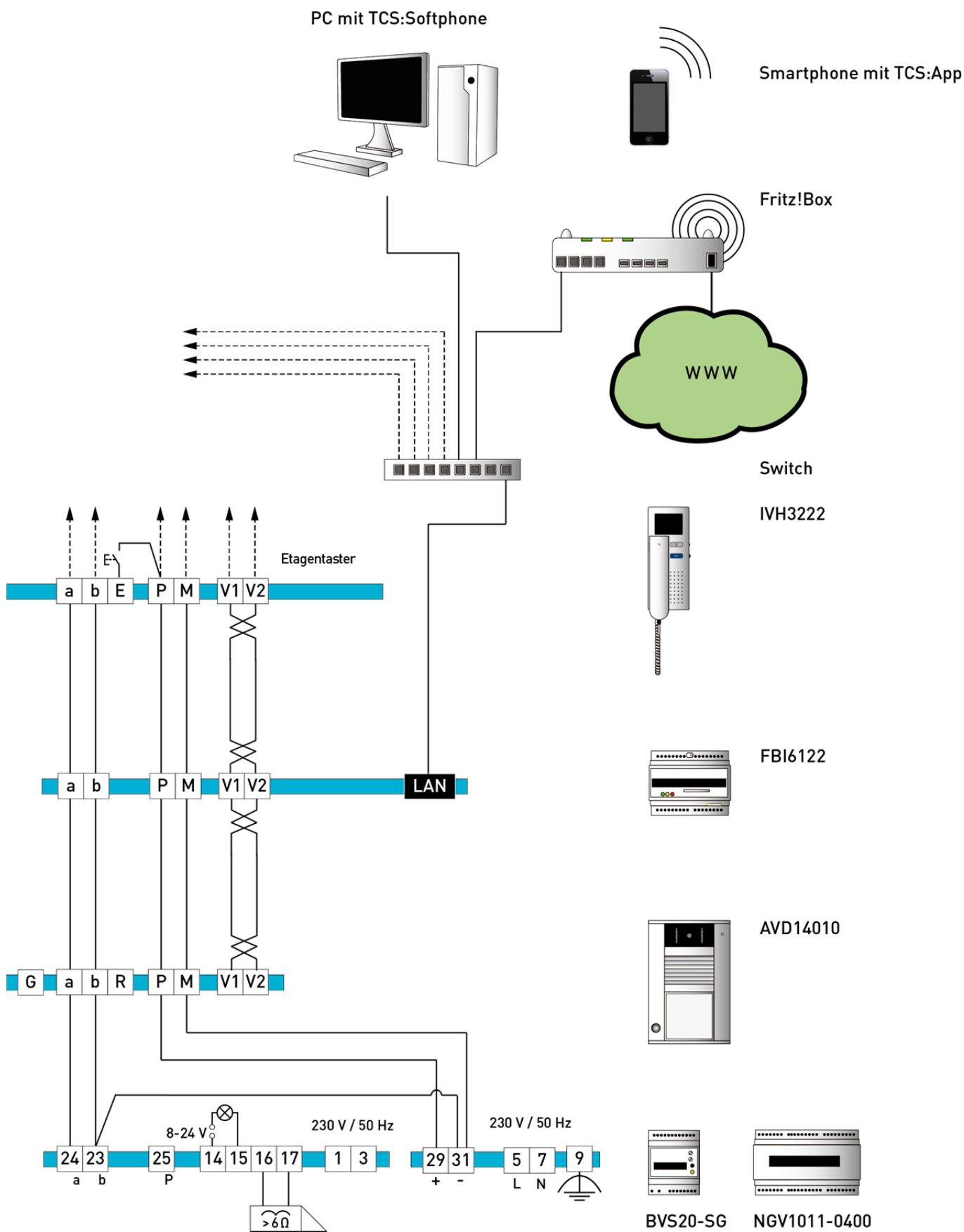
Abb. 6: Schaltungsbeispiel
