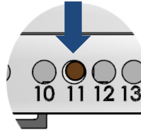
Abb. 9: Werkseinstellung laden
