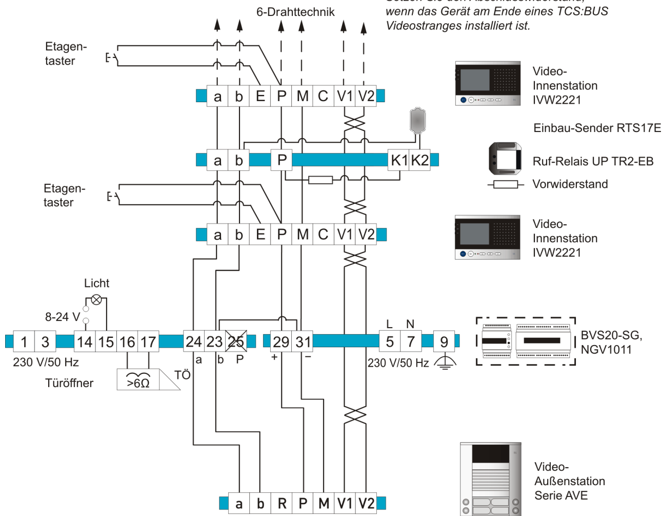
Abb. 3: Schaltungsbeispiel
