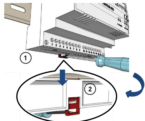
Abb. 3: Demontage von der Hutschiene
