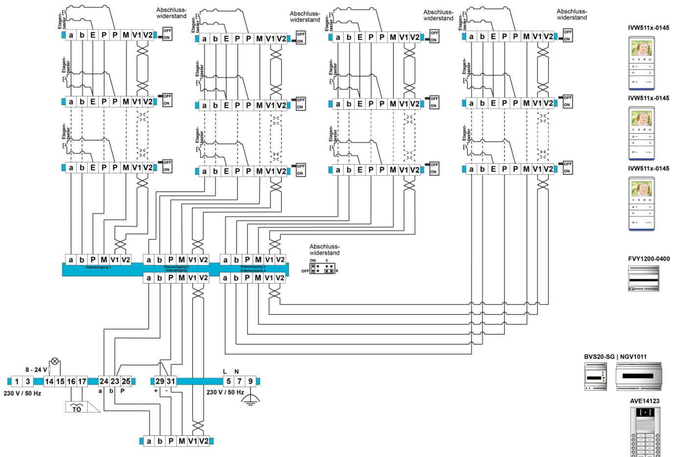
Abb. 4: Schaltungsbeispiel
