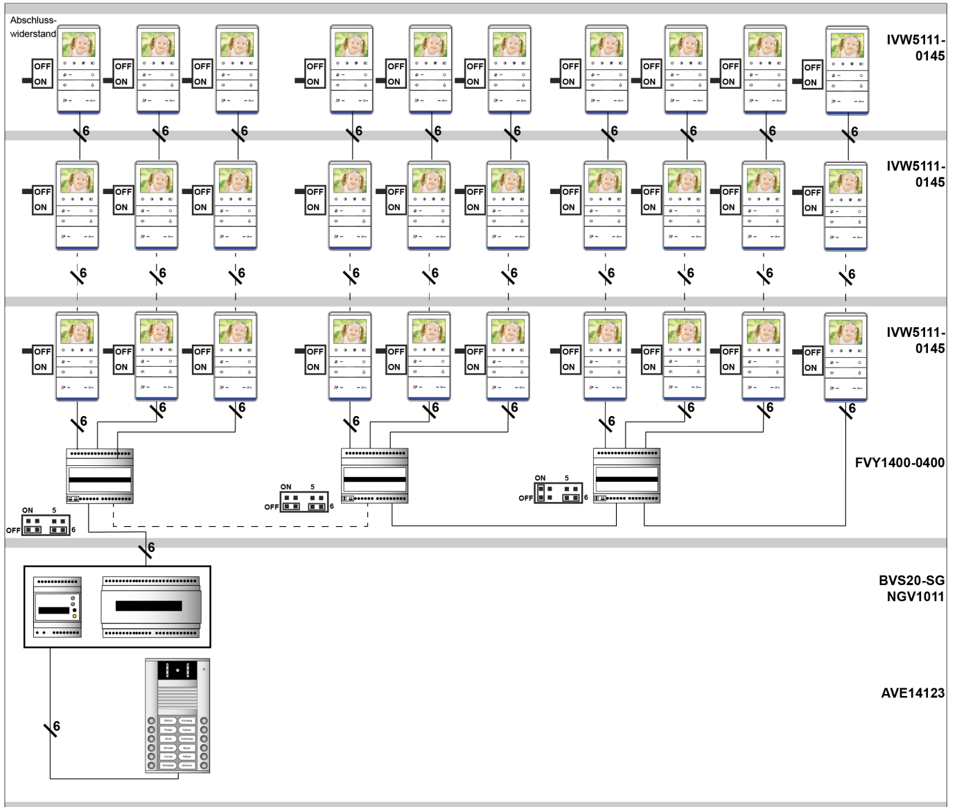
Abb. 5: Prinzipbild
