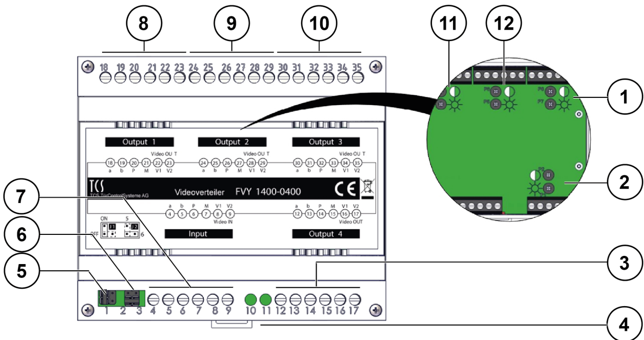
Abb. 1: Geräteübersicht
