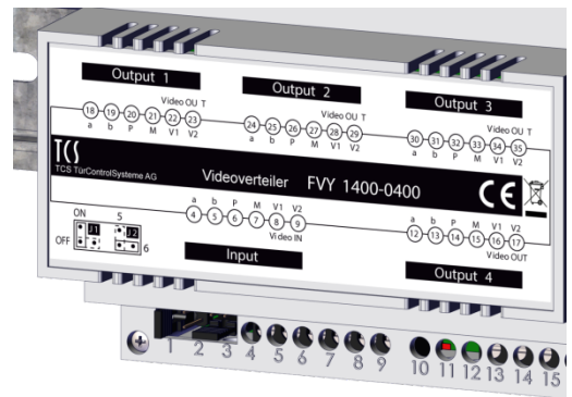
Abb. 3: Beschriftung Anschlüsse
