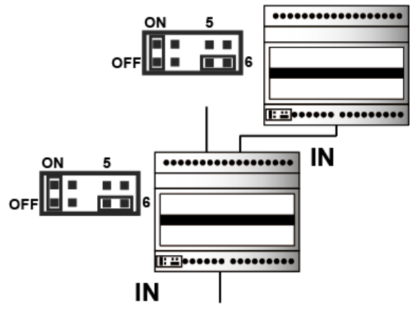
Abb. 7: Prinzipbild Reihenschaltung
