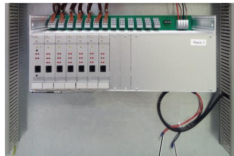
Abb. 8: Batterien anschließen
