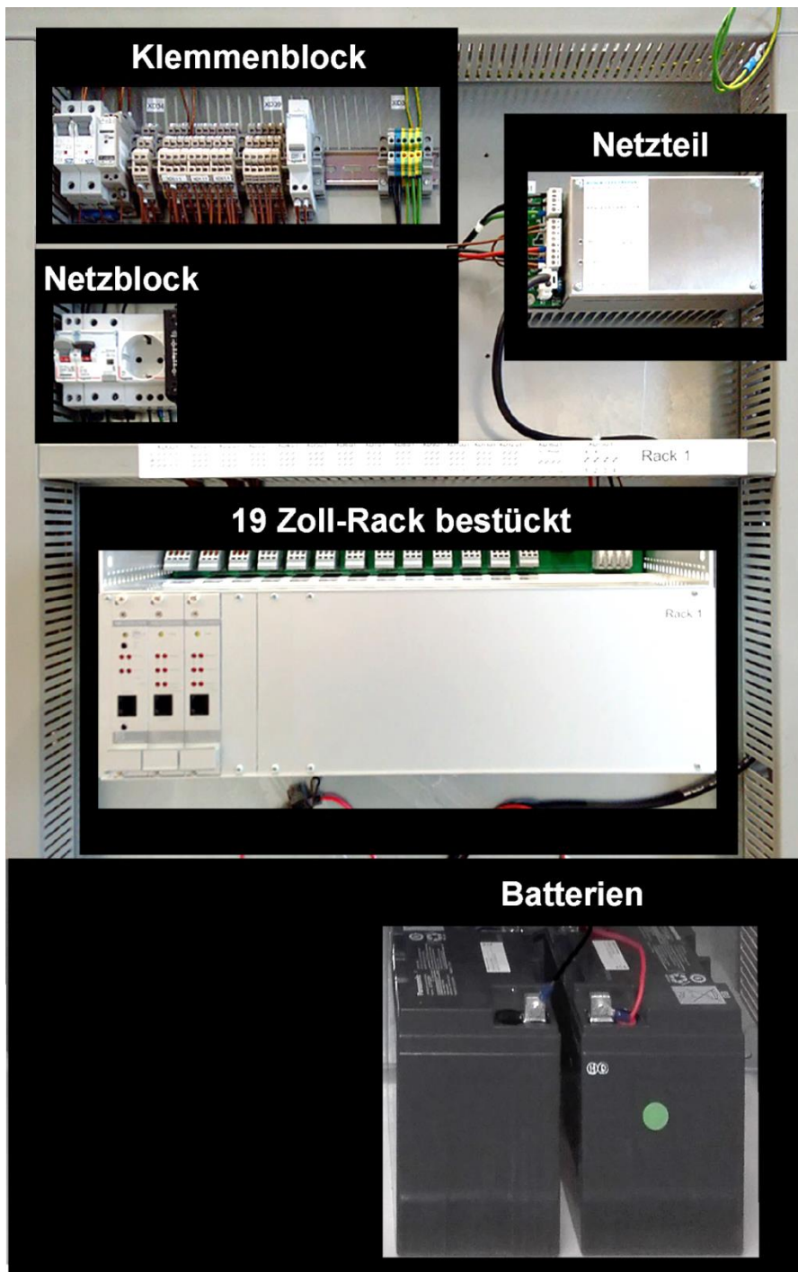
Abb. 1: Bestückungsübersicht Montageplatte
