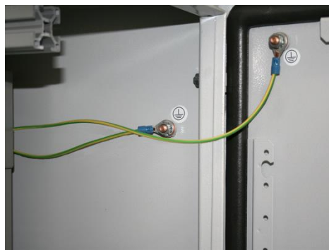
Abb. 3: Anschlüsse Schutzschrankwand und Schutzschranktür
