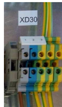
Abb. 4: Klemme Schutzleiteranschluss
