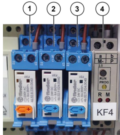
Abb. 12: Fehlblock
