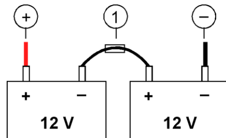
Abb. 7: Batterien anschließen
