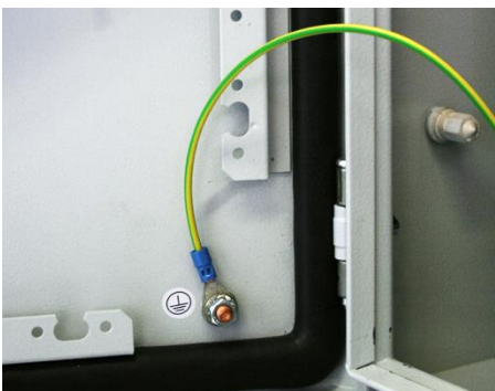
Abb. 2: Anschluss einer Schutzschranktür
