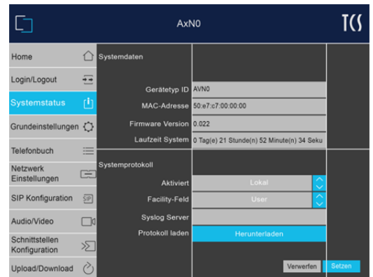
Abb. 12: Menü Systemstatus
