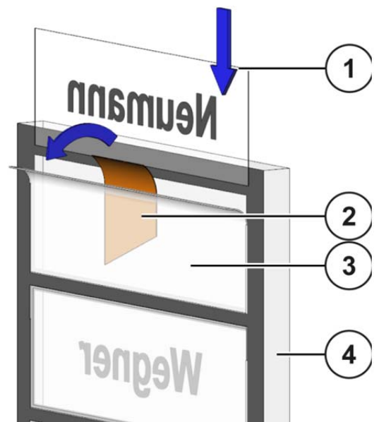
Abb. 8: Namensschild einstecken
