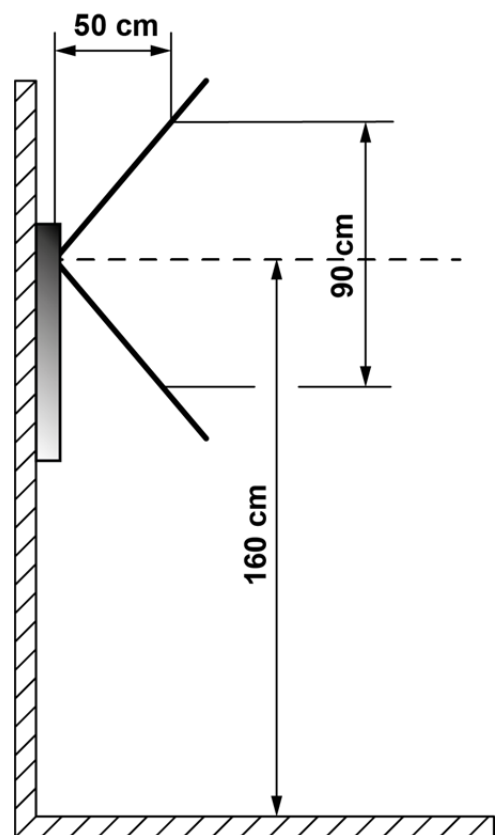
Abb. 1. Montagehöhe
