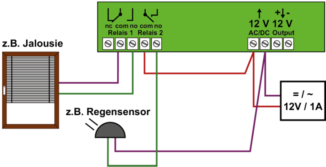
Abb. 11: weitere Anschlussmöglichkeiten
