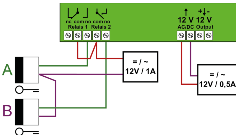
Abb. 10: getrennte Stromversorgung
