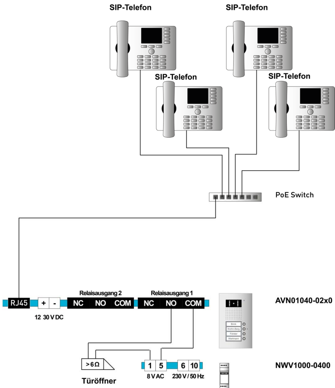
Abb. 9: Schaltungsbeispiel
