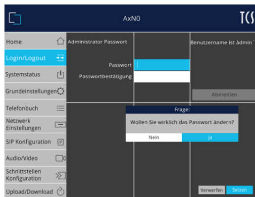
Abb. 11: Menü Login/Logout
