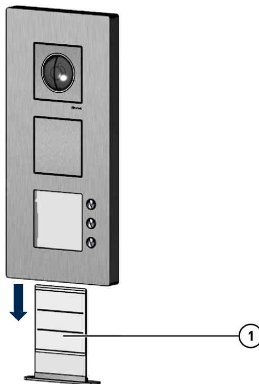
Abb. 3: Namensschildträger entfernen
