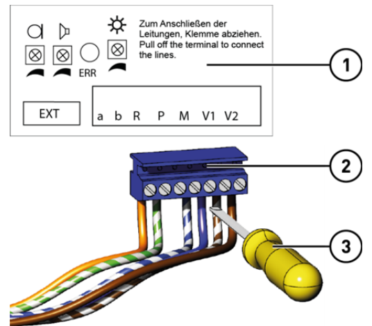
Abb. 7: Leitungen Anschließen
