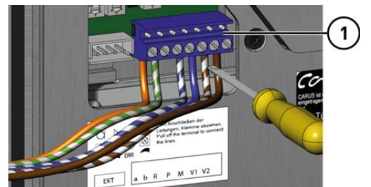
Abb. 8: Anschlussklemme aufstecken
