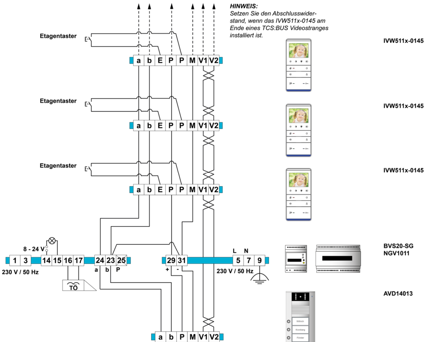
Abb. 9: Schaltungsbeispiel
