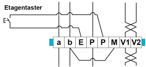
Abb. 8: 5-Drahttechnik
