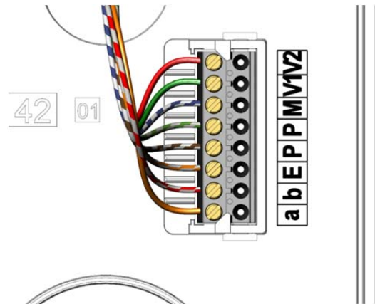
Abb. 5: Leitungen anschließen
