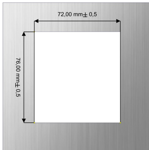
Abb. 1: Größe Frontplattenausschnitt
