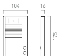
Video-2-Draht Außenstation Serie AVC
