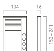
Außenstation Serie PAK
