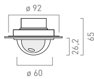
Dome-Kamera zur Unterputzmontage
