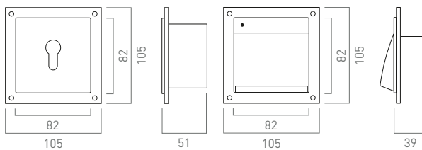
Schlüsselschaltermodul Beleuchtungsmodul
