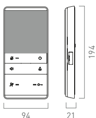
Mit TASTA Montageschale Audio
