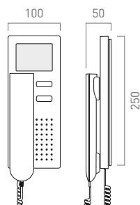
Video-2-Draht Türtelefon
