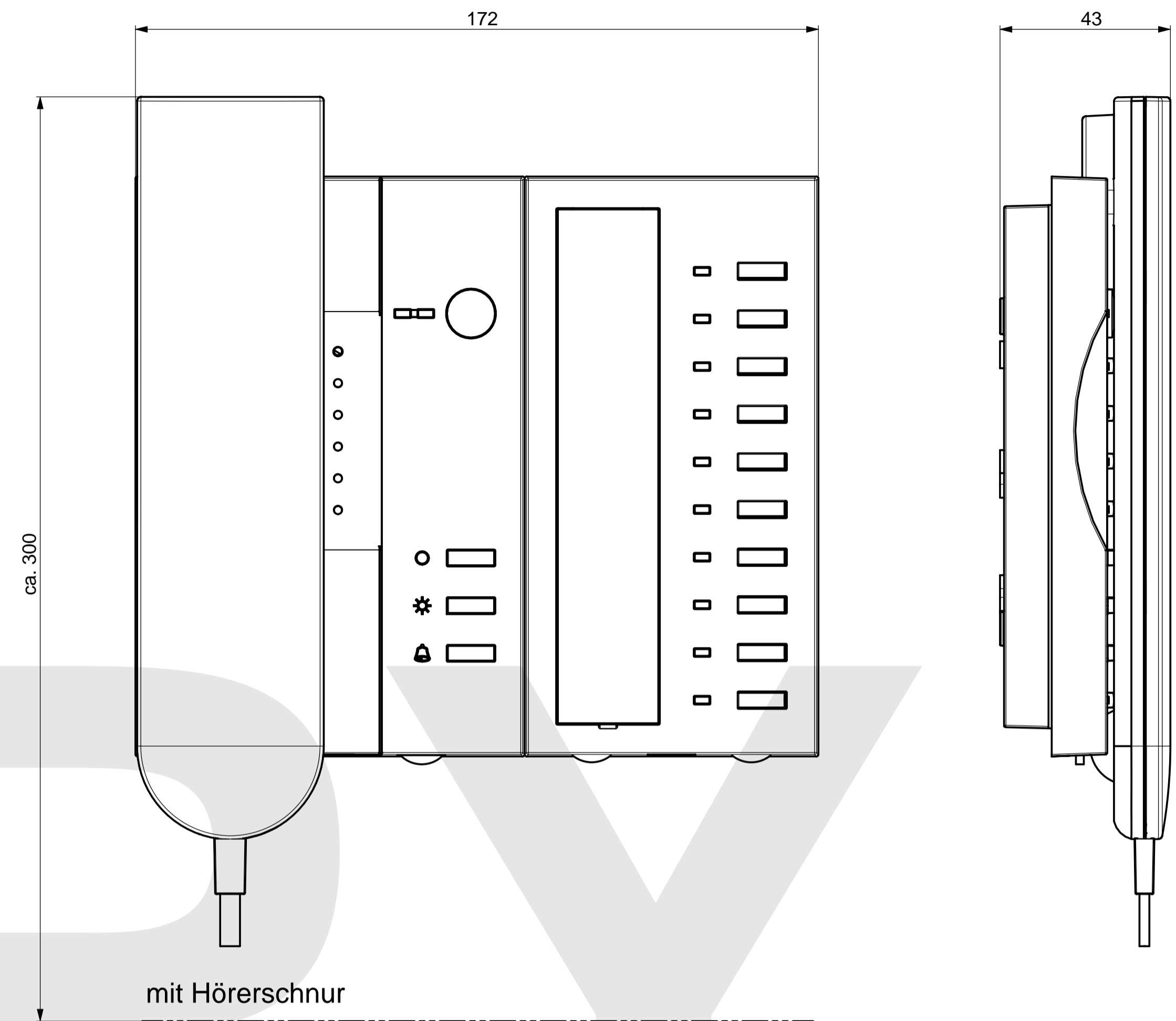
Montageansicht
