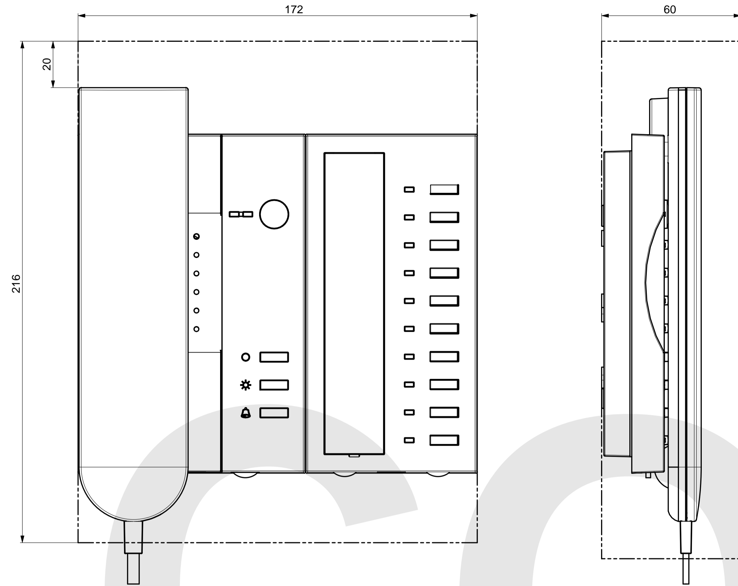
Gehäusemaß
