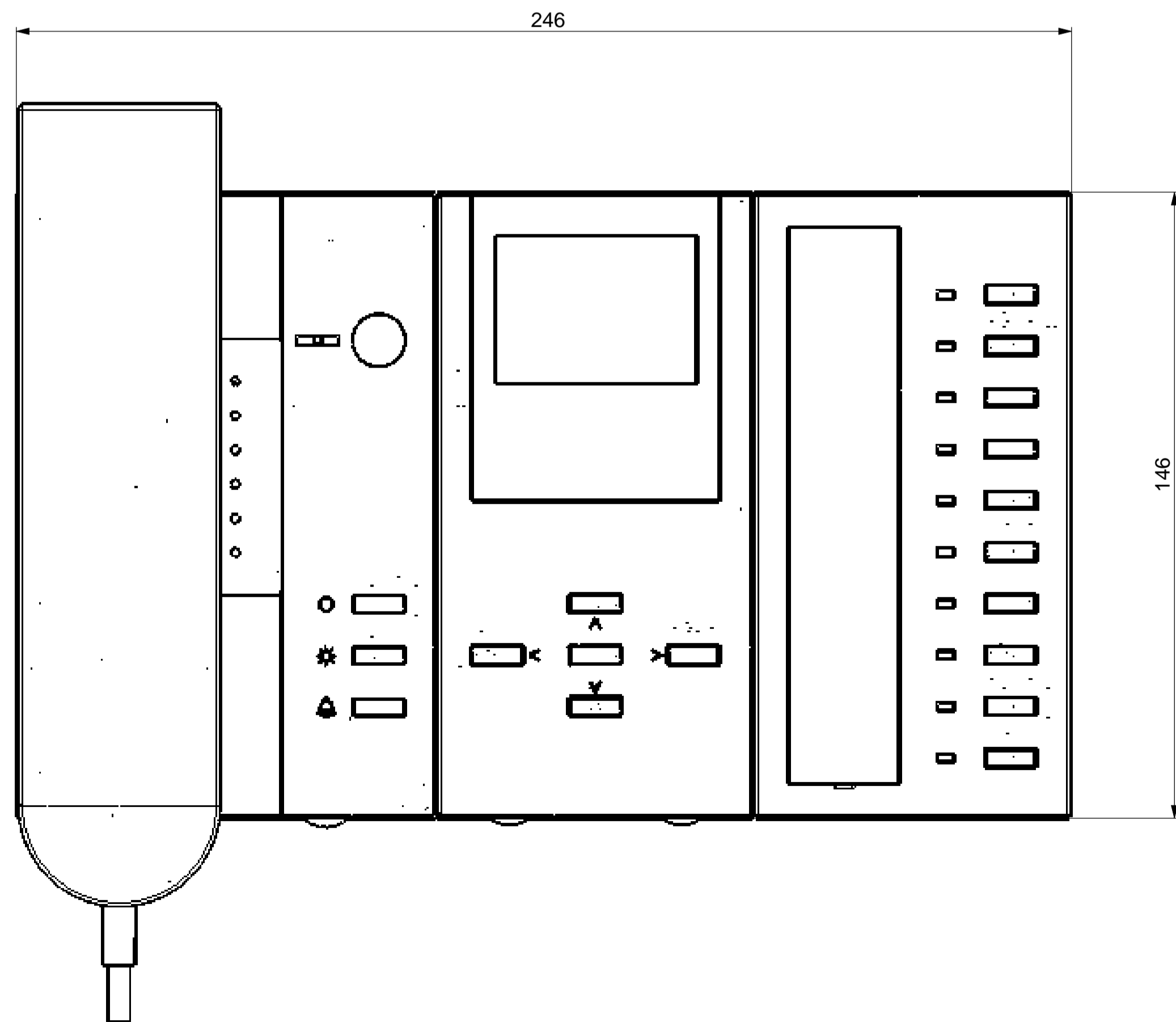
Gehäusemaß
