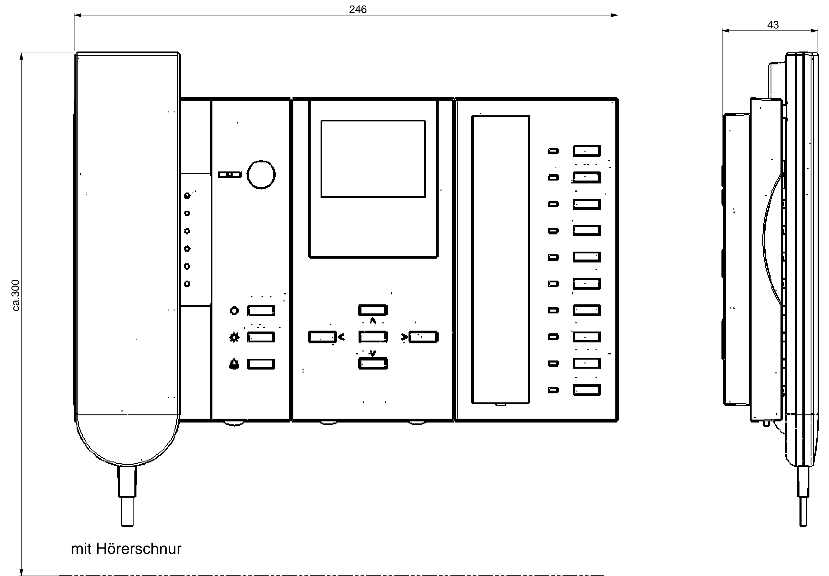
Montageansicht
