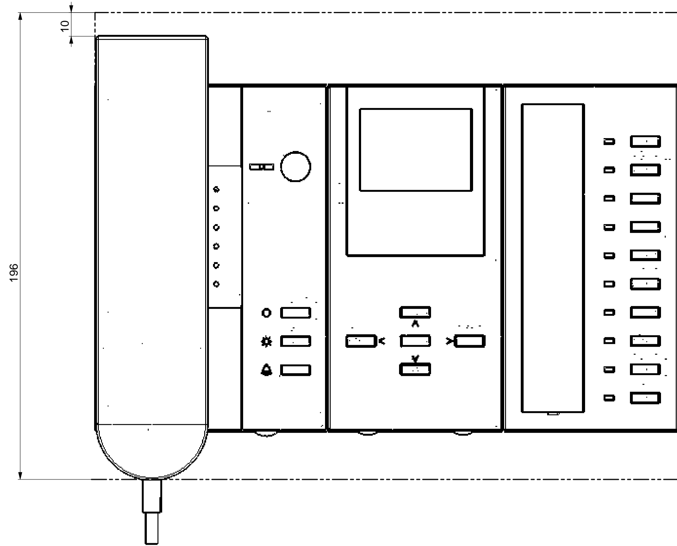
Gehäusemaß
