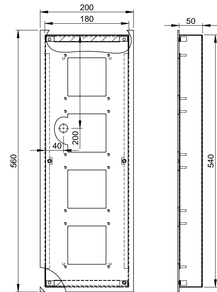
ZAU2004-0030 Unterputzmontageset mit 4 Ausschnitten, 1-spaltig
