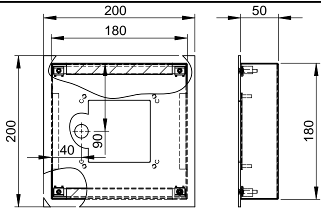
ZAU2001-0030 Unterputzmontageset mit 1 Ausschnitt
