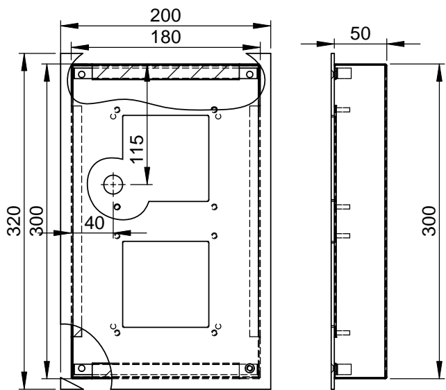
ZAU2002-0030 Unterputzmontageset mit 2 Ausschnitten, 1-spaltig
