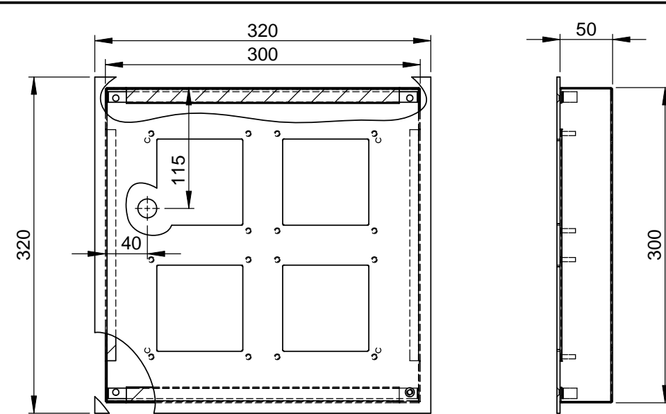
ZAU2007-0030 Unterputzmontageset mit 2 x 2 Ausschnitten, 2-spaltig
