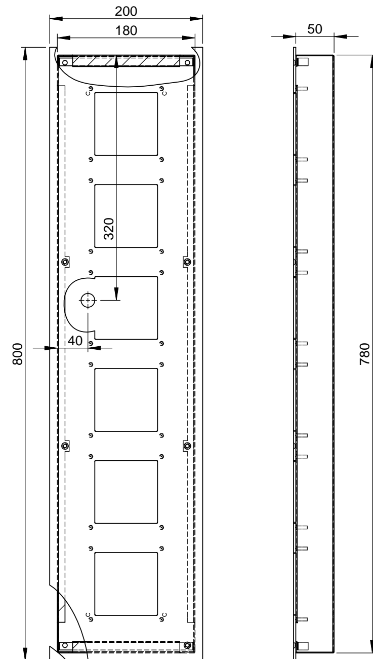
ZAU2006-0030 Unterputzmontageset mit 6 Ausschnitten, 1-spaltig
