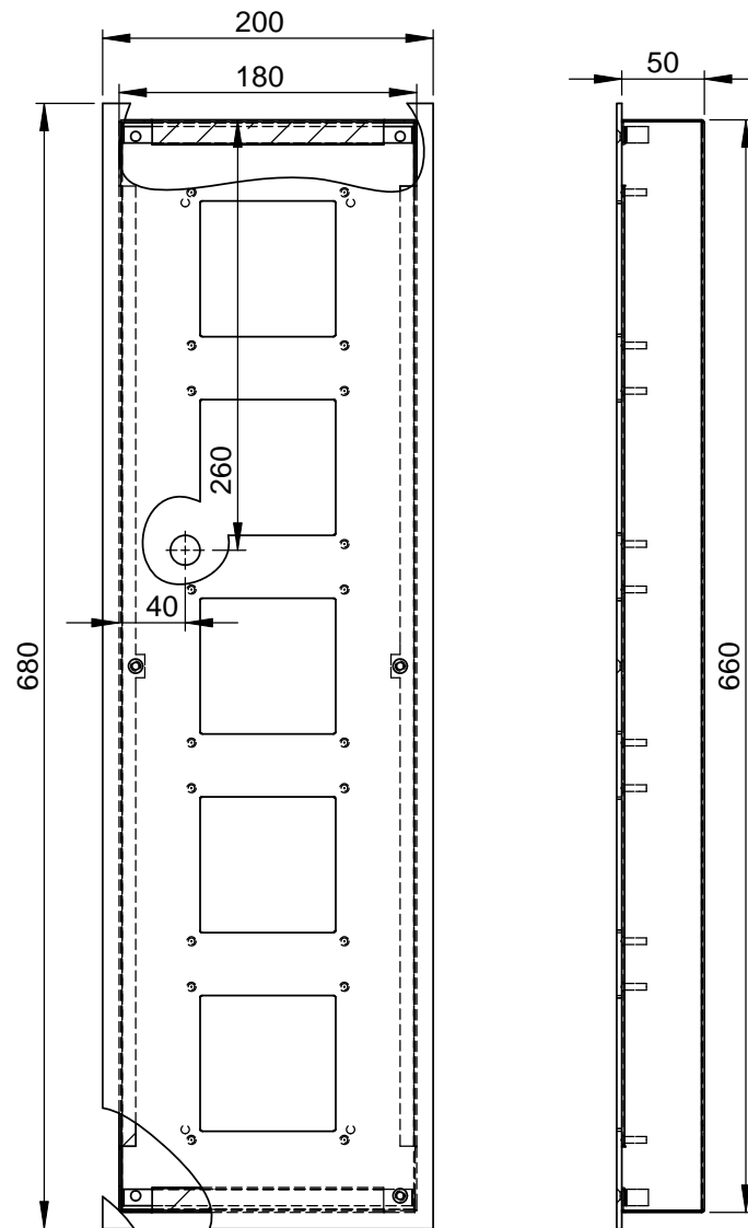
ZAU2005-0030 Unterputzmontageset mit 5 Ausschnitten, 1-spaltig
