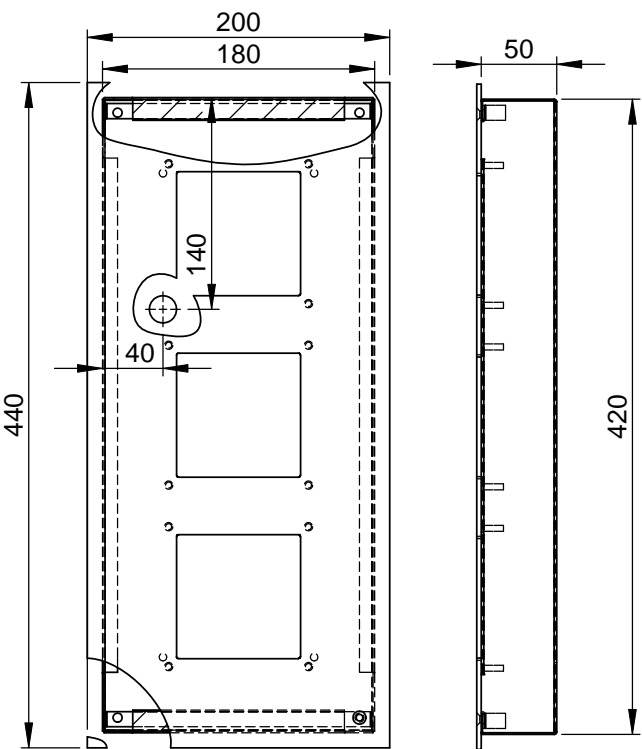
ZAU2003-0030 Unterputzmontageset mit 3 Ausschnitten, 1-spaltig
