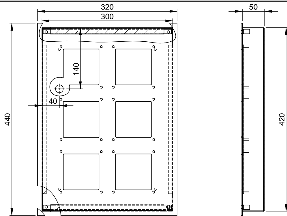
ZAU2008-0030 Unterputzmontageset mit 2 x 3 Ausschnitten, 2-spaltig
